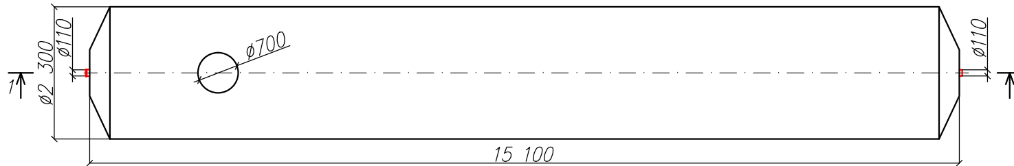
Вид сверху
