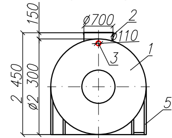
Вид спереди
