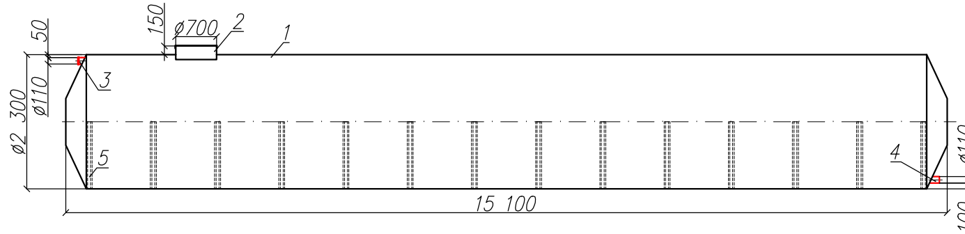
Разрез 1-1
